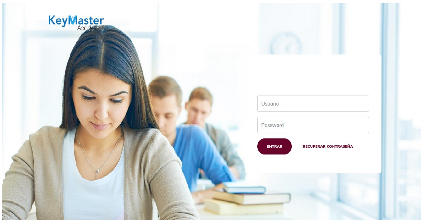
Figura 5: Login.
