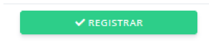
Figura 15: Registrar.
