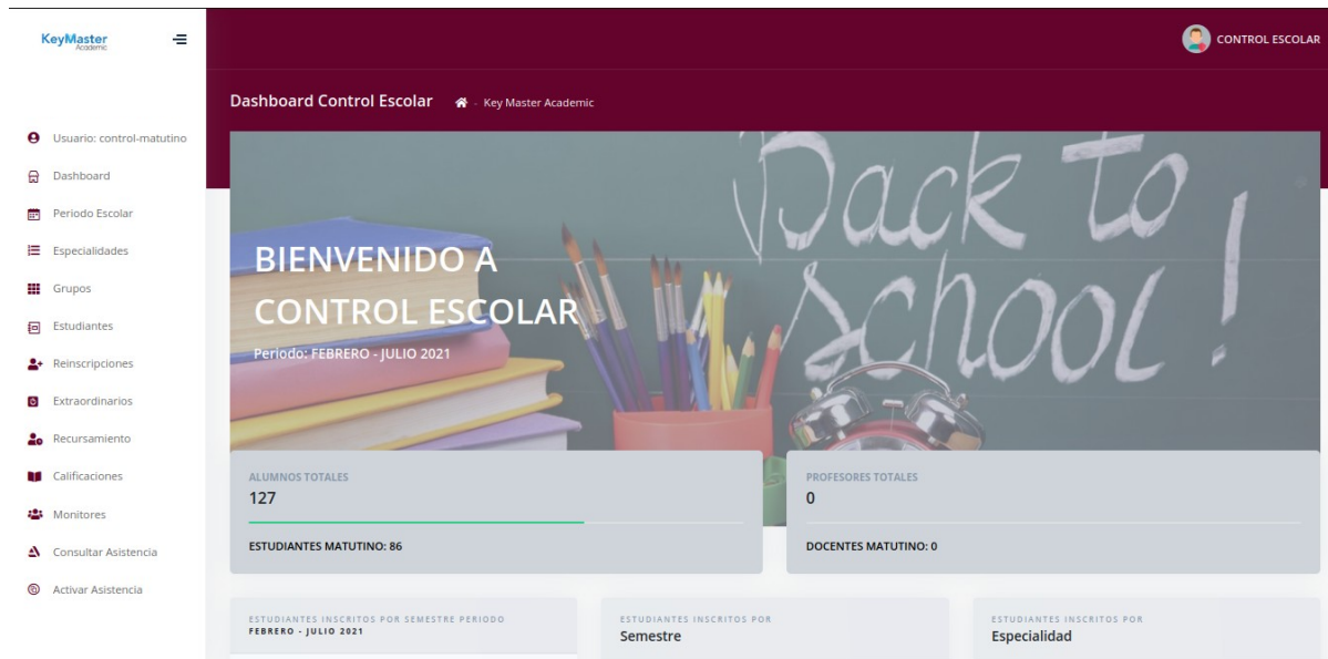
Figura 8: Vista.
