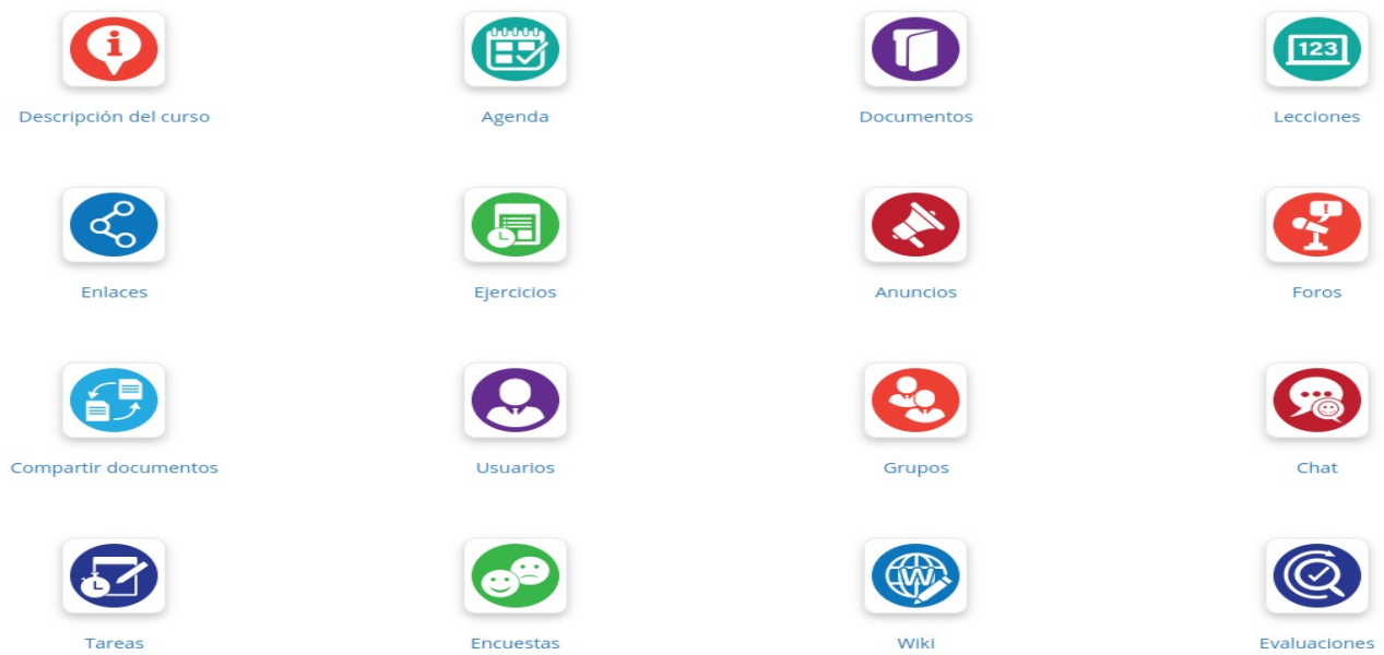
Figura 5: Opciones.
