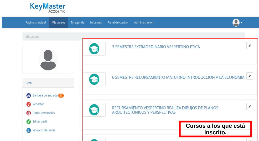
Figura 4: Curso.
