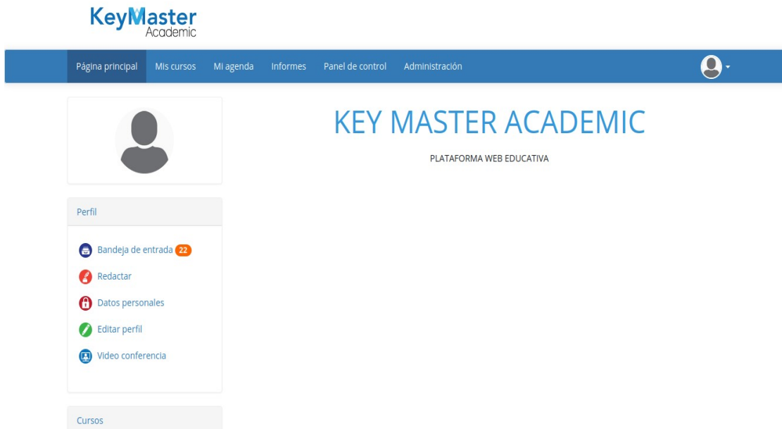
Figura 2: Pantalla principal.
