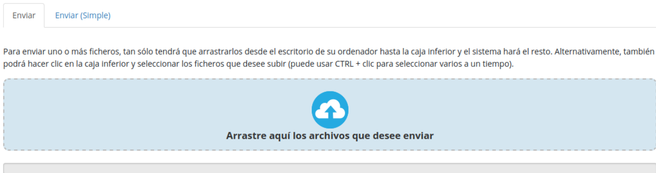
Figura 10: Archivos.
