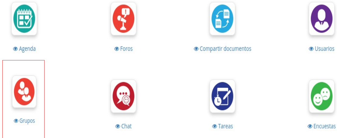
Figura 5: Grupos.
